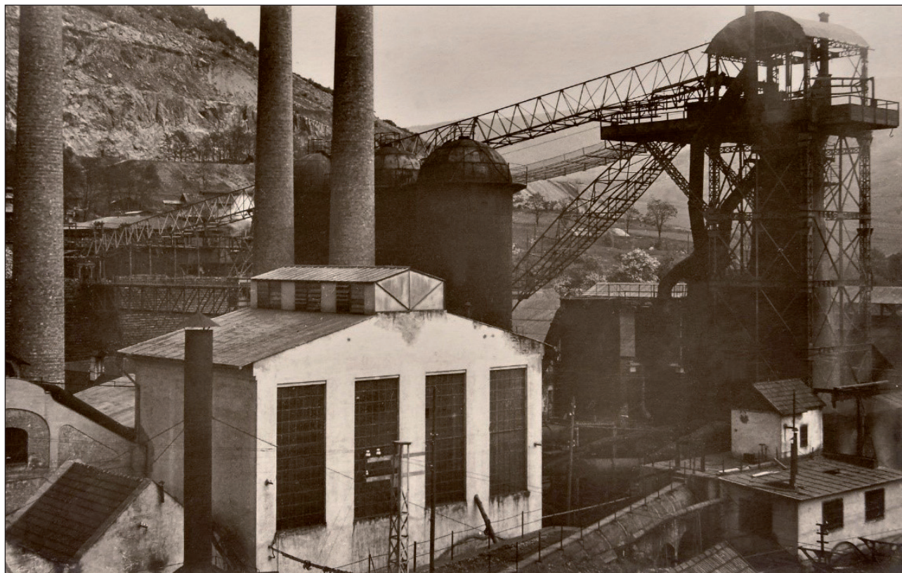
Vysoká pec v Tisovci bola v roku 1935 prestavaná na obsah 245 m 3 s výkonom 140 ton surového železa za 24 hodín (Zdroj: Archív O. Laudára)
